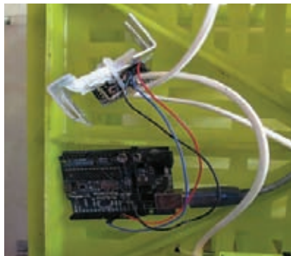
Электроника робота
