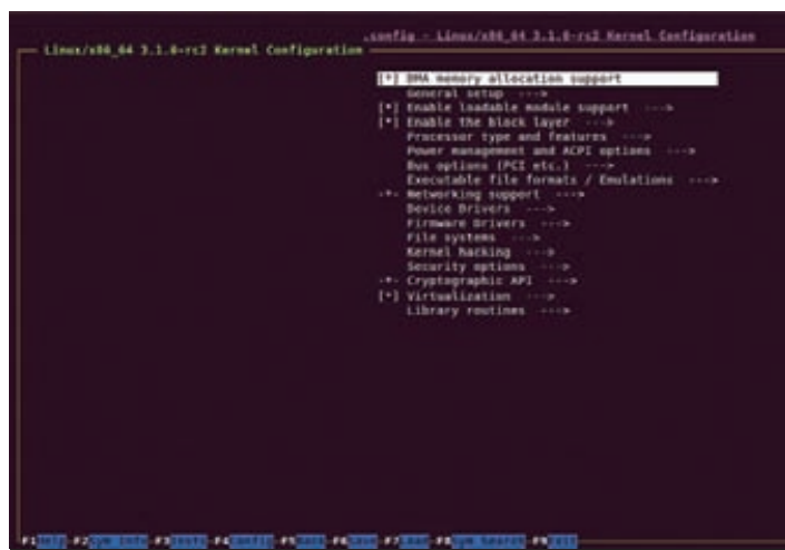
Обновленный menuconfig
