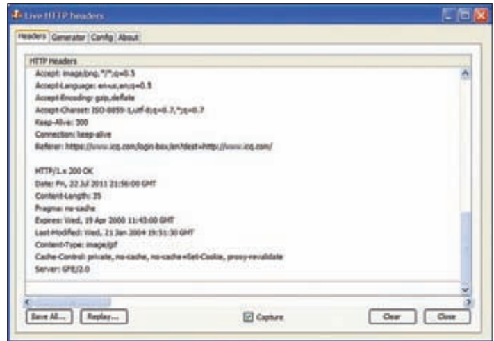
Плагин LiveHTTPHeaders
