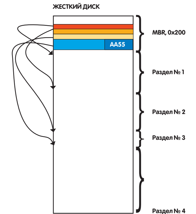
Схема разбиения жесткого диска на разделы с помощью MBR
