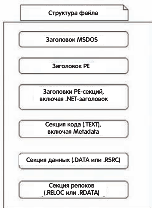
Схема .NET исполняемого файла
