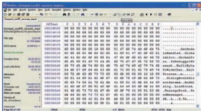
Список импортируемых API-функций виден невооруженным глазом
