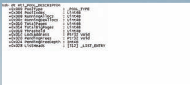
Структура POOL_DESCRIPTOR
