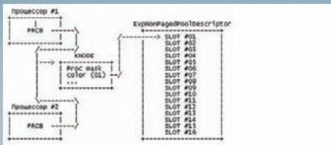
Описание пула при нескольких процессорах
