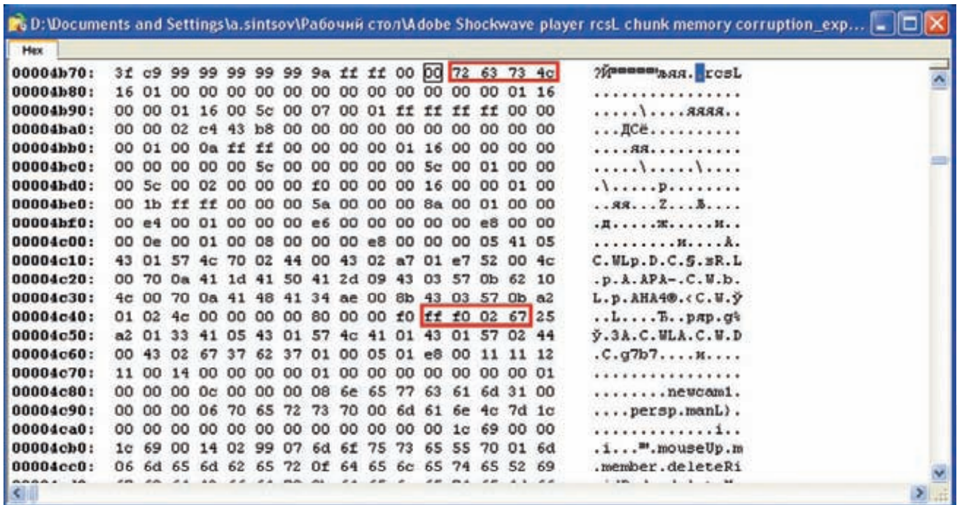
Формат DIR. rcsL-блок и данные, влияющие на EAX
