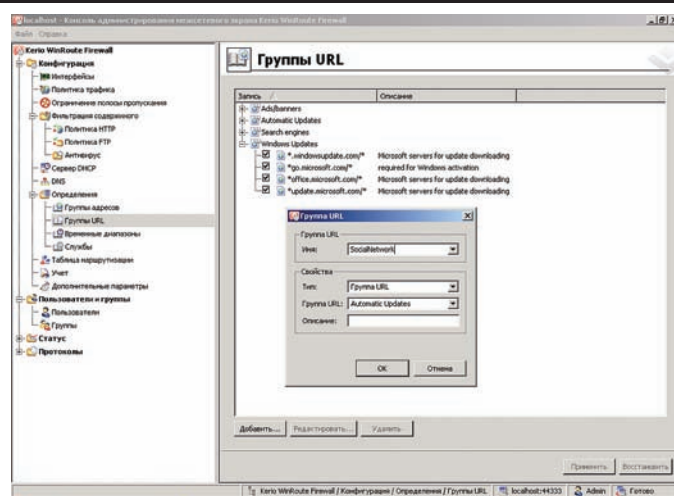
Создаем группу URL в Kerio WinRoute
