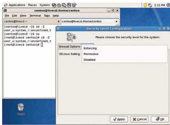
Выбор режима работы SELinux
