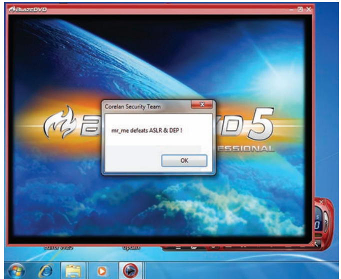
BlazeDVD. Результат открытия плейлиста
