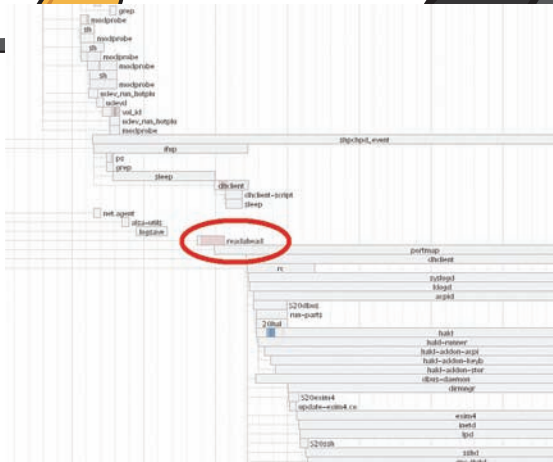
Readahead в графике bootchart
