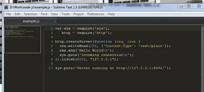
Пример асинхронного веб-сервера
