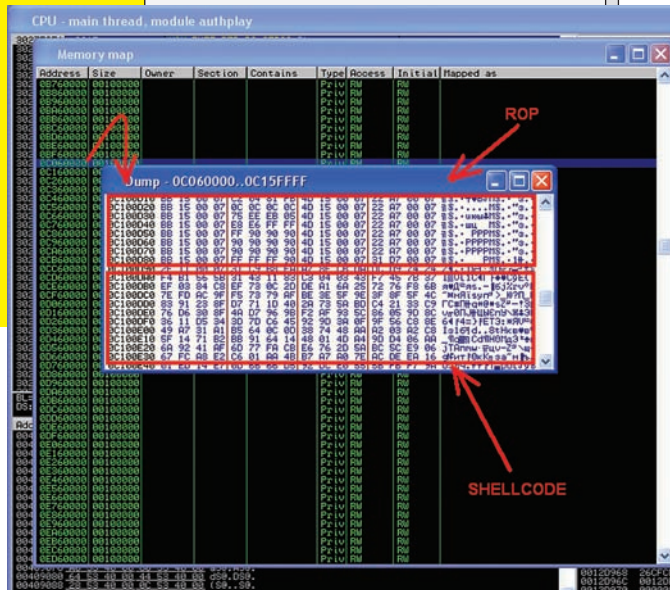
Acrobat Reader. Содержимое heap-spray
