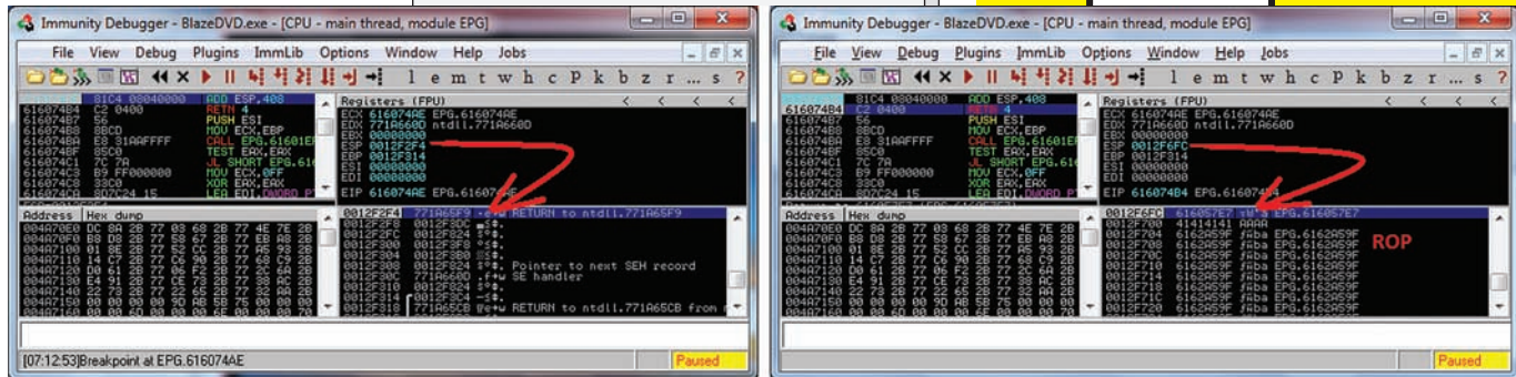
BlazeDVD. «Обработчик» восстанавливает стек для работы ROP
